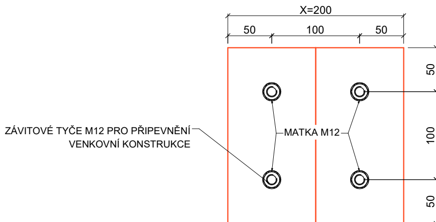
POHLED PŘEDNÍ
