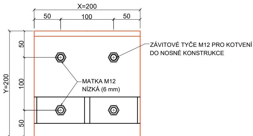
POHLED ZADNÍ
